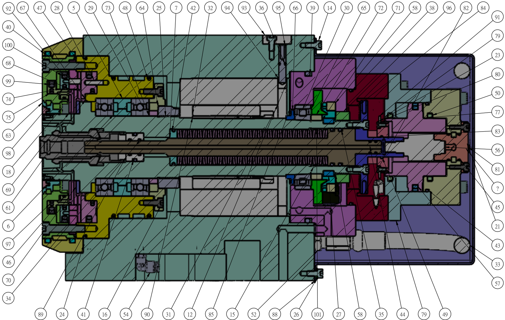
剖面圖 B-B 比例 1 : 2.5
